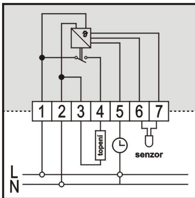
zapojení MTU2
